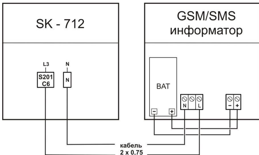
Рис. 2 Подключение питающей электросети от прибора SK-712
