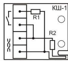
Плата Контроля Шлейфа-1
