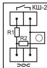
Плата Контроля Шлейфа-2
